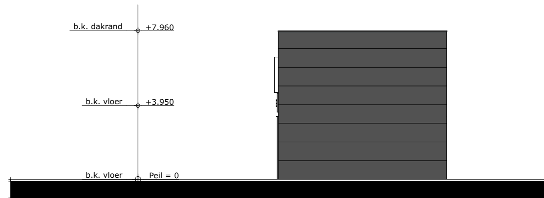
ZUID-OOSTGEVEL
