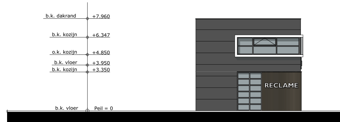
NOORD-WESTGEVEL
