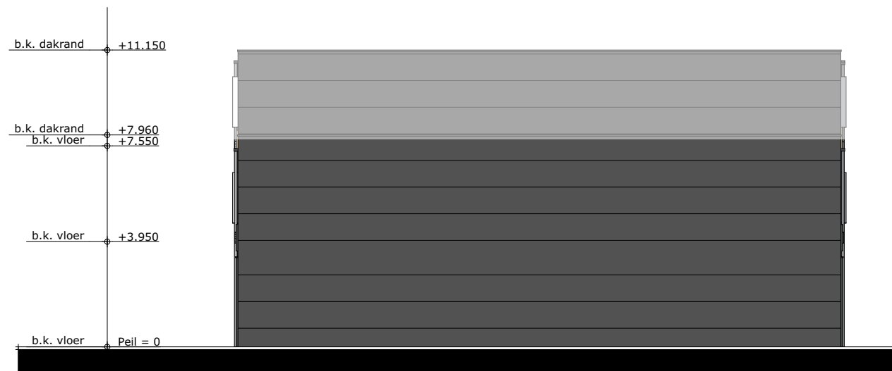
ZUID-OOSTGEVEL
